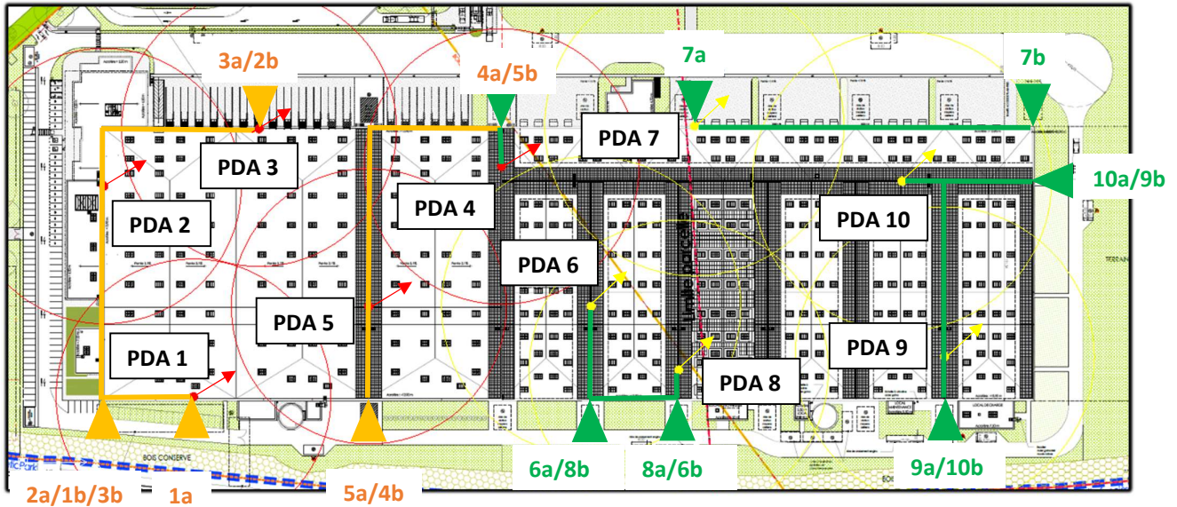
Implantation des paratonnerres, conducteurs de descente et prises de terre.
